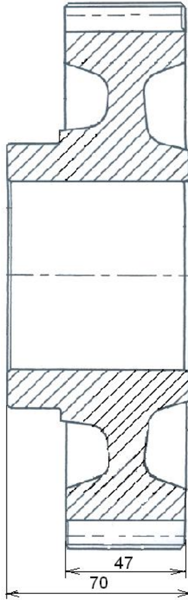
Рис. 1. Шестерня 2-ой передачи 239.1701050-10 Было
