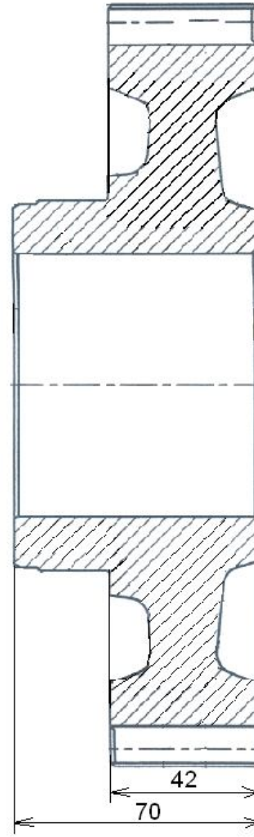
Рис. 2. Шестерня 2-ой передачи 1509.1701050 Стало
