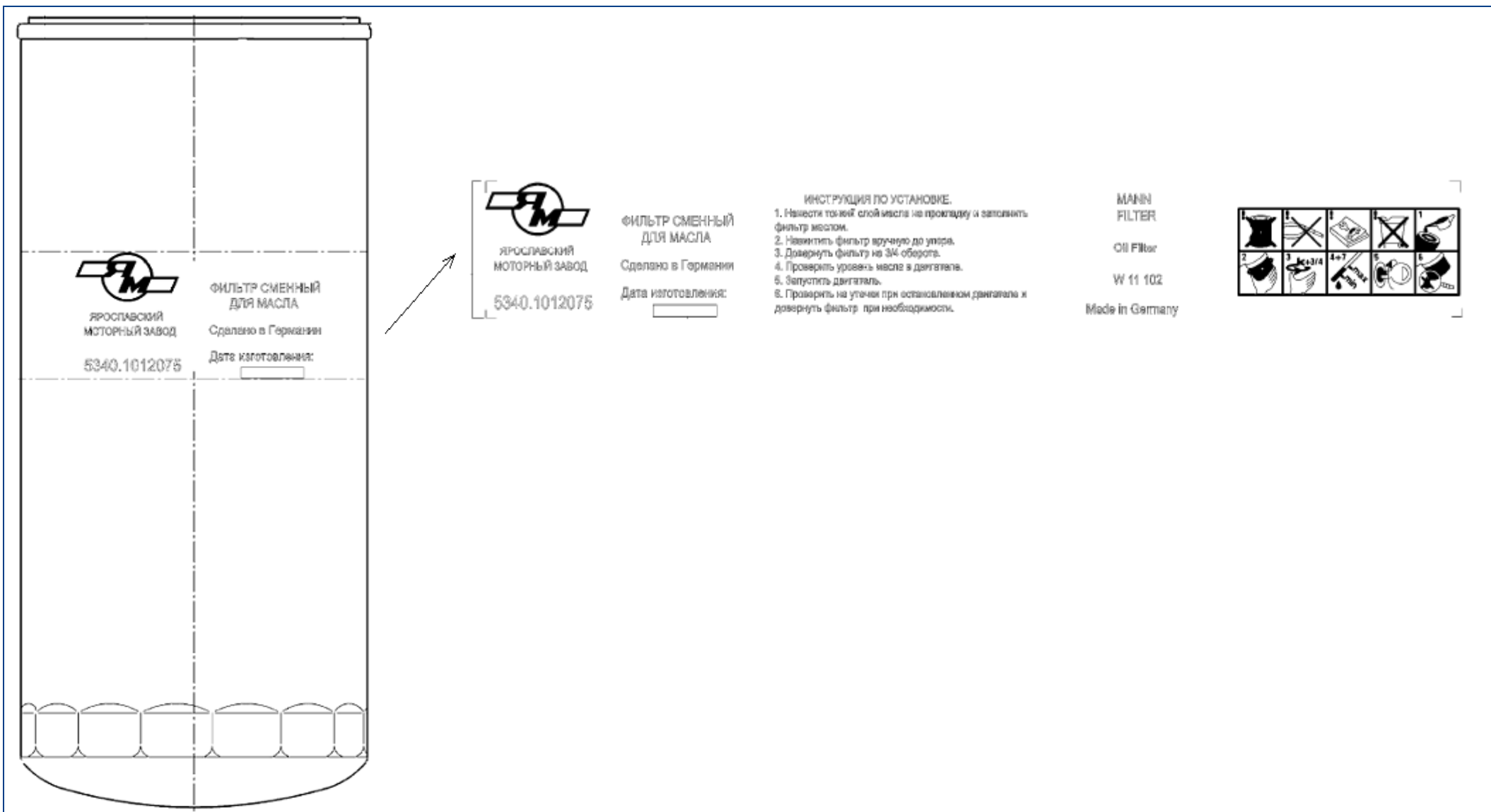
Рис 4. Фильтр сменный для масла 5340.1012075 (W 11 102)
