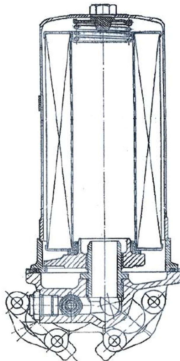
Рис. 2 Фильтр очистки масла 238Б-1012010-Б2
