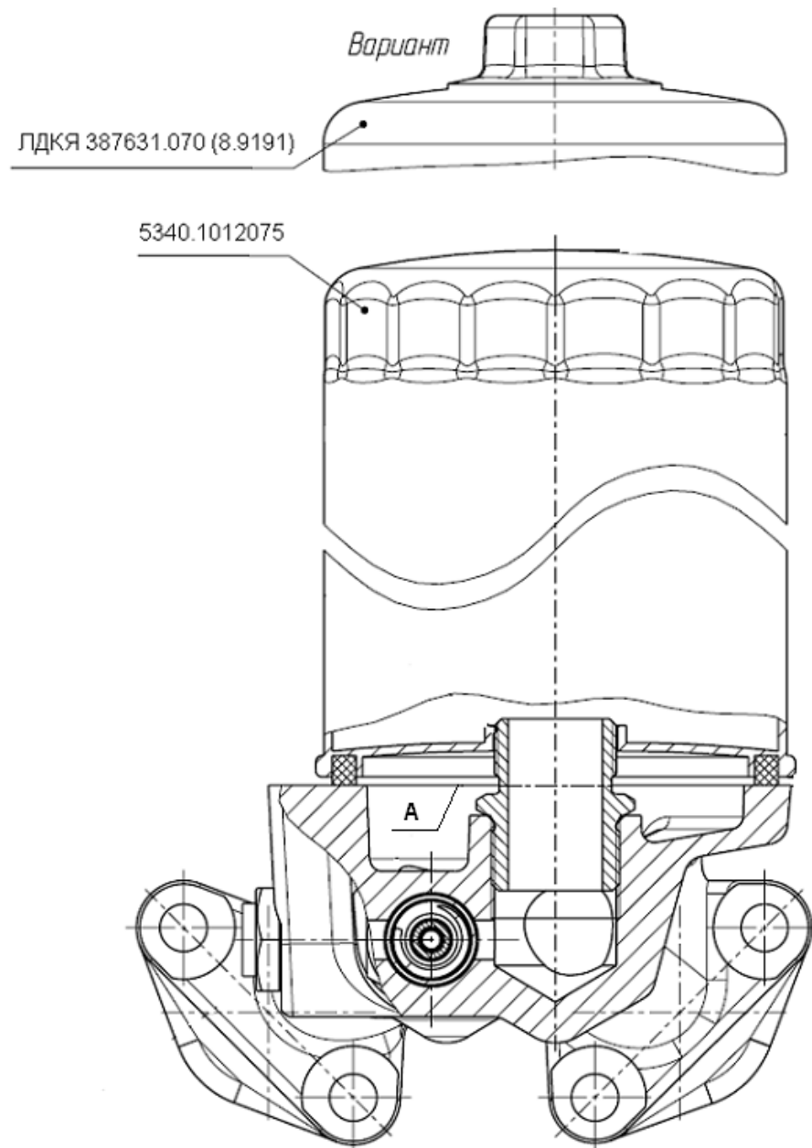
Рис. 1 Фильтр очистки масла 658.1012010
